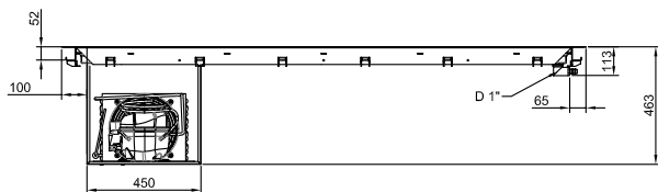
Boční
